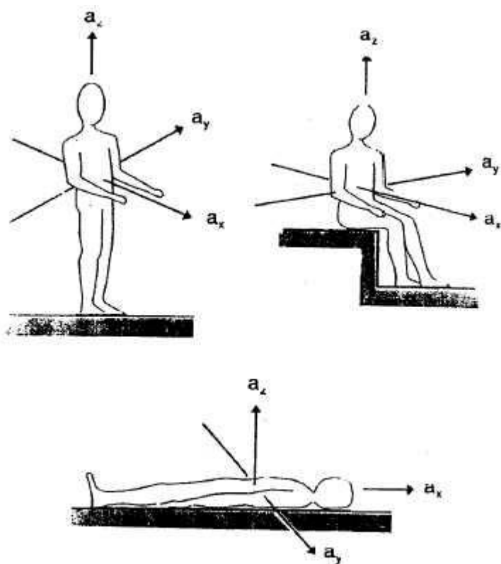
Figura 3: Sistema de coordenadas biodinámicas para medir las aceleraciones (adaptado según ISO 2631). ax, ay, az = aceleración en la dirección de los ejes, x, y, z; eje x dirección espalda-pecho; eje y dirección derecha-izquierda; eje z dirección pies-cabeza.
